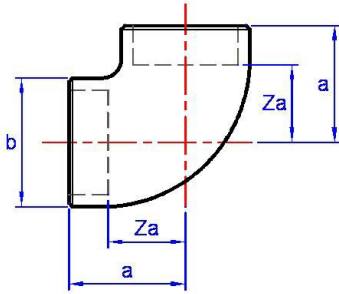
12GHD Elbow
