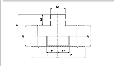
YP25 Tee
